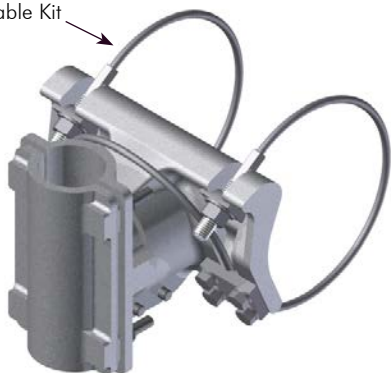
AB-0280/ AB-0320 Cable Kit
