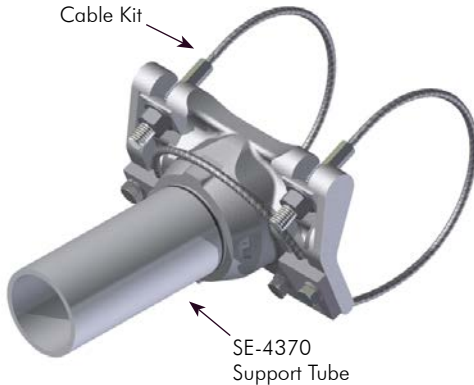
AB-0280/ AB-0320 Cable Kit
